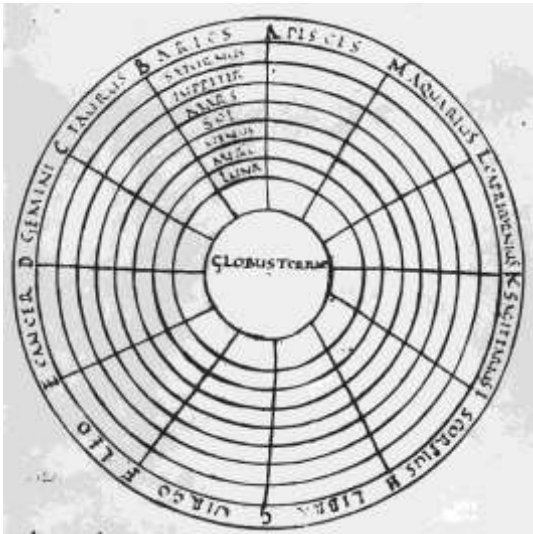
Једна од најранијих представа геоцентричног система која је дошла до нас (латински приказ Макробија: «Коментар на Сан Сципиона» рукопис IX век)
